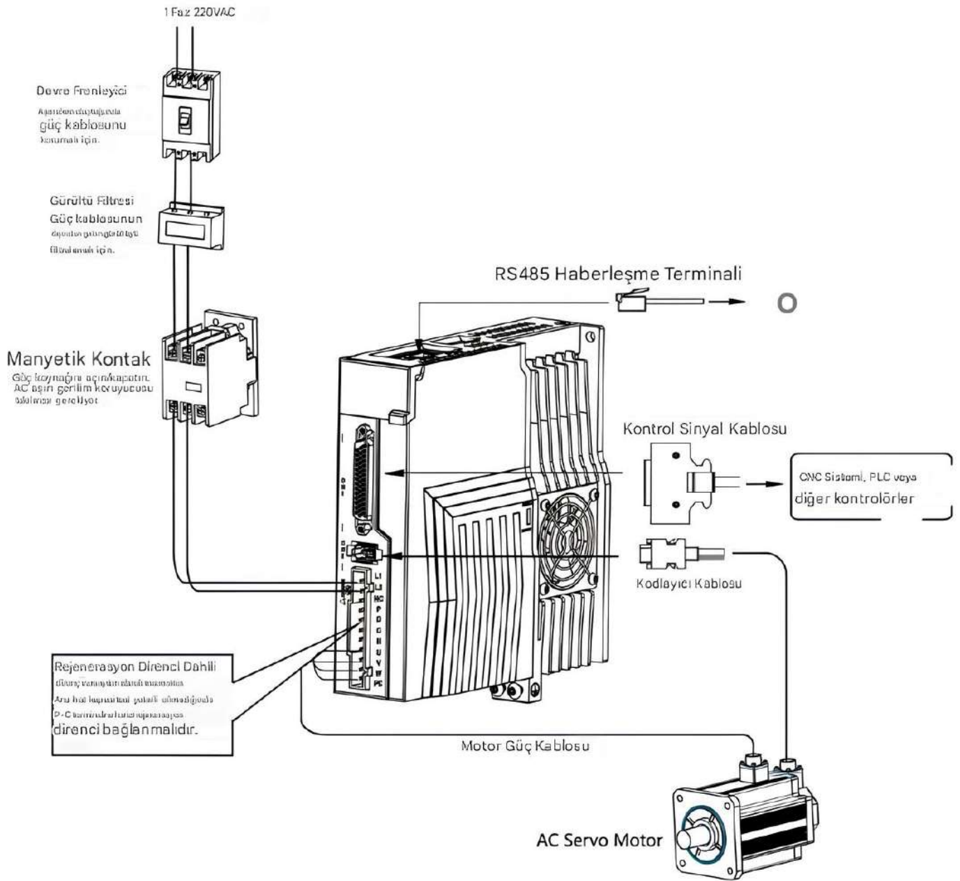
Resim 4.1 Servo Sistem Kablolaması
